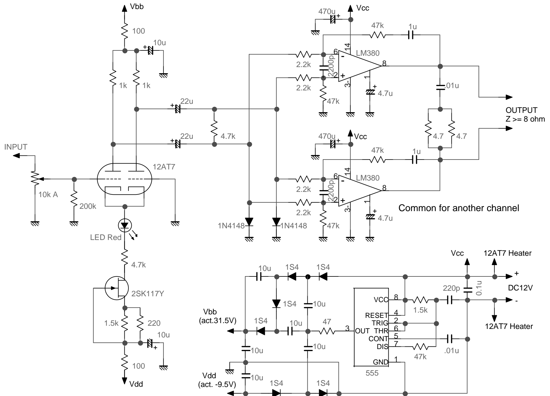
12AT7-LM380 Full-Balance AMP. 2020.1.26 A.Sakai
