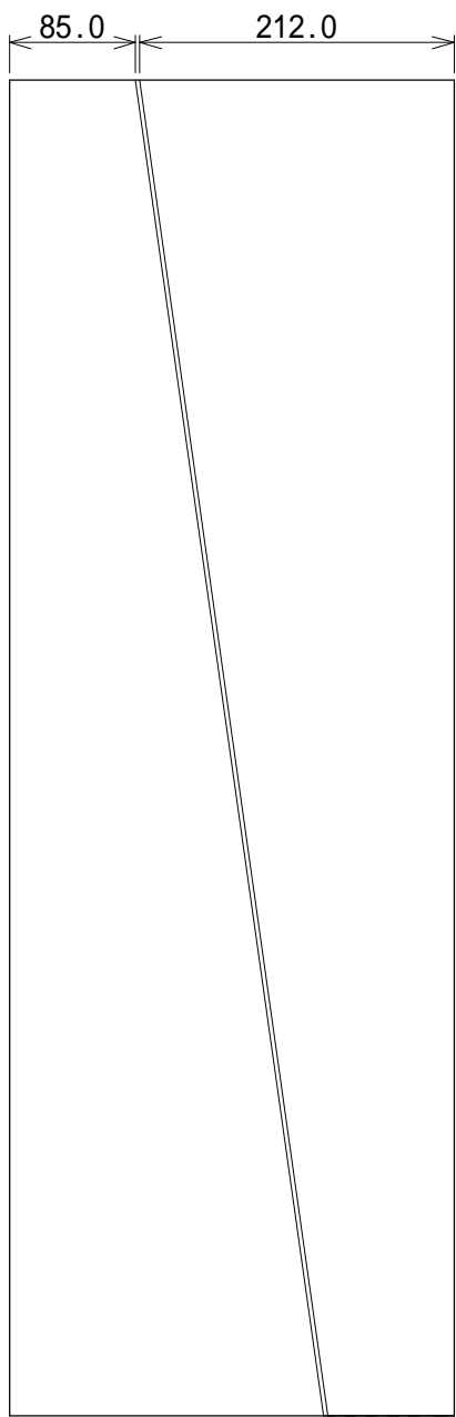
側板 (X2) 18tパイン集成材 300X900mm
